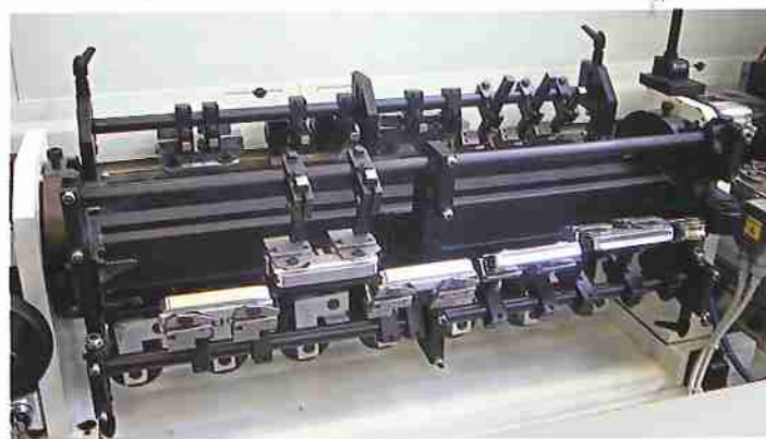
Cambio settori di pressione a revolver Cambio sectores de presión a revolver
