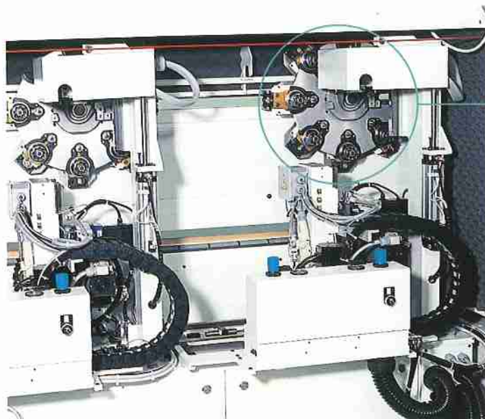
Gruppo arrotondatore- spigolatore 2 motori con cambio utensili automatico
