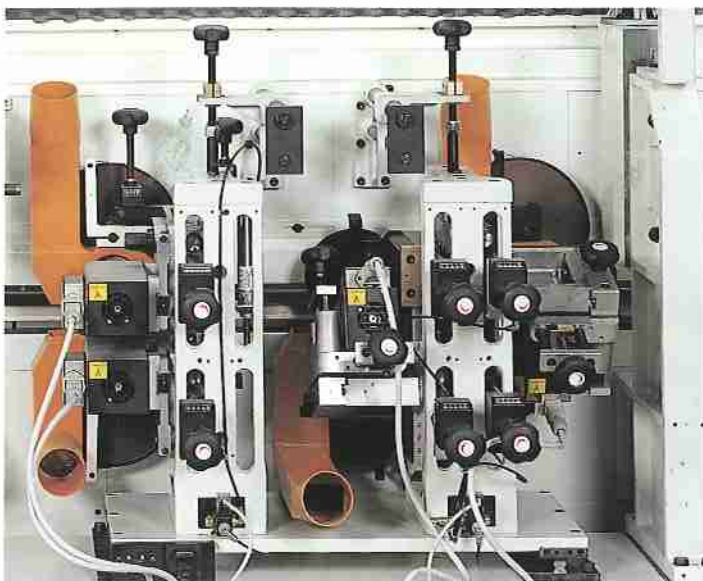
Gruppo spigolatore Grupo biselador
