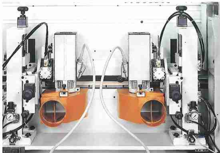
Gruppo toupie Gruppo tupi para ranuras
