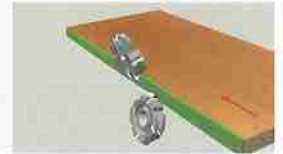
Gruppo rifilatore- spigolatore Fine trimming unit Groupe d'affleurage de finition Bündigfräs-/ Fein Radiusfräsaggregat Grupo refilador- biselador
