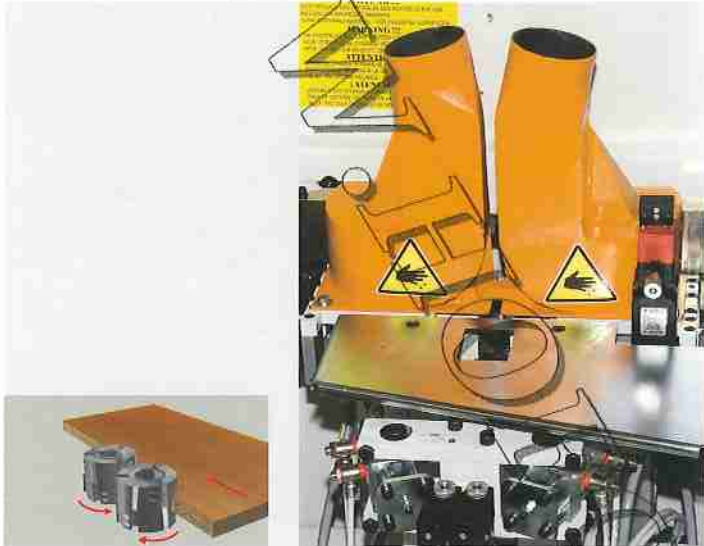
Gruppo rettificatore Pre-milling unit Groupe rectifieur Fügefräsaggregat Grupo rectificador
