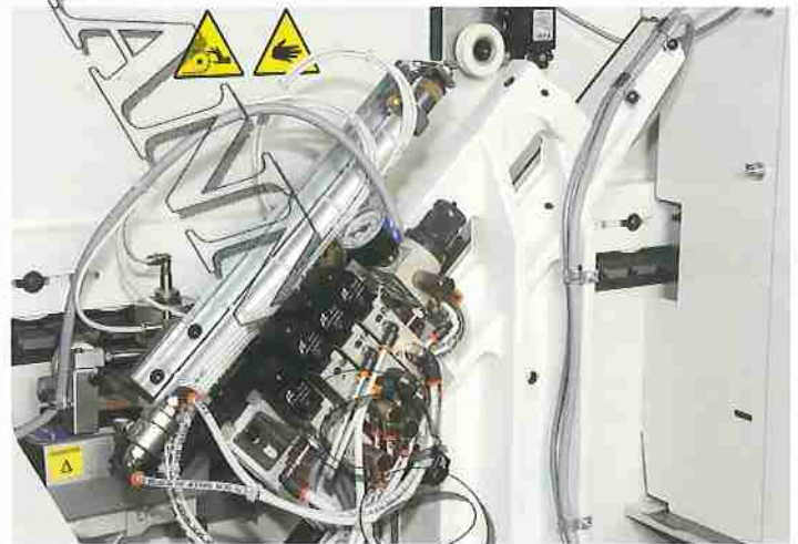
Gruppo traseatore End-trimming unit Groupe de coupe en bout Kappaggregat Grupo retesteador
