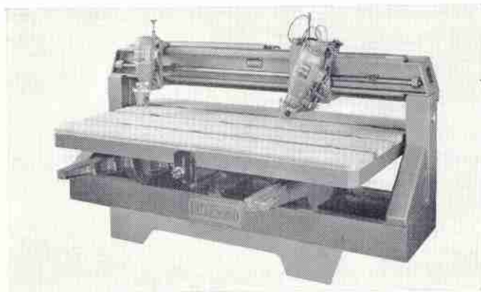
Automatische luftgesteuerte Türenfräse Typ DOF für Lichtausschnitte sowie Briefkasten- und Ventilations-schlitzte, schrägstellbarer Kopf
