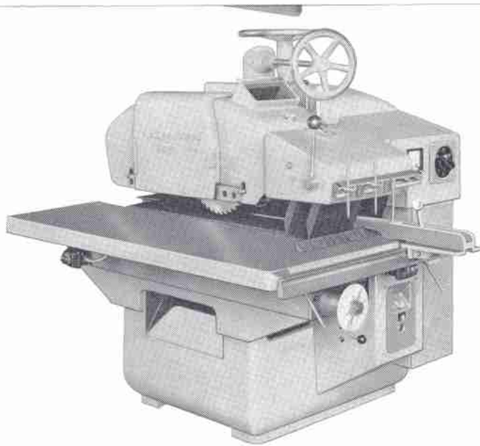
Automatische Besäum-, Zuschneide- und Vielblattkreissägen mit Plattenbandvorschub · Plattenbandbreite 160 bis 300 mm · 4 Baugrößen mit Motorleistungen von 7,5 bis 75 PS · Sonderausrüstungen zum Schneiden kurzer Hölzer · Abgebildet ist Modell CR 1
