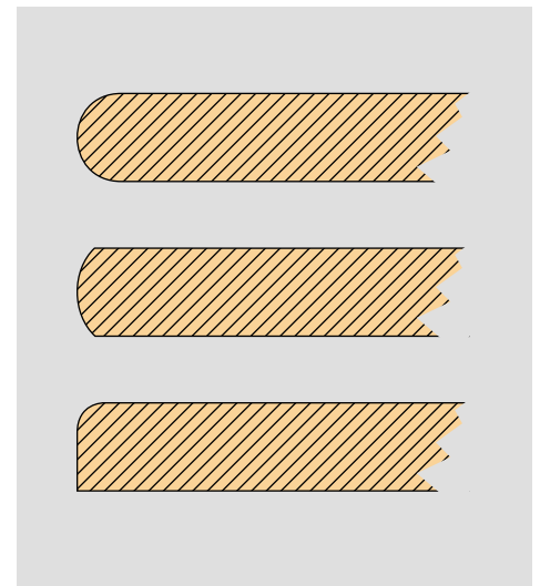
Beispiele möglicher Kantenprofile Examples of possible edge contours
