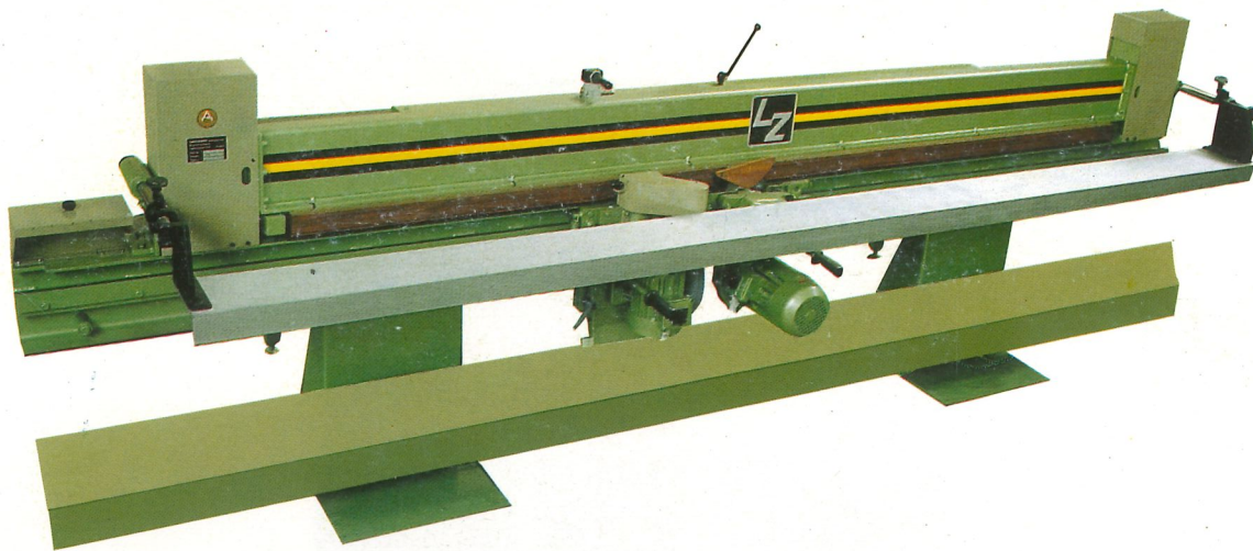
Fräsaggregat im Einsatz auf einer LZ 2 mit beweglichen Abnahmetisch. Jointing device in use on a LZ 2 with movable front table.
