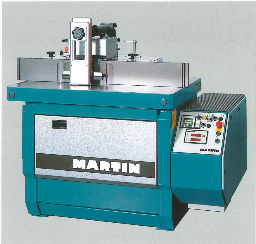
MARTIN Starrfräse T 20 mit Schutzvorrichtung Centrex T 2000 und der stufenlosen Drehzahlregelung T 2003
