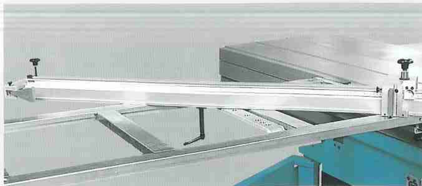
T 782 A fixe Gradeinteilung am Quertisch
