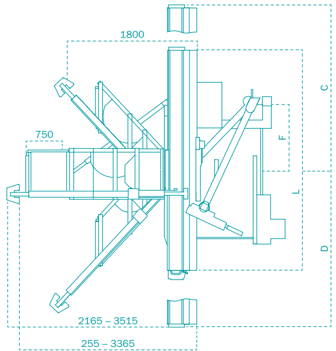
T75 | Draufsicht
