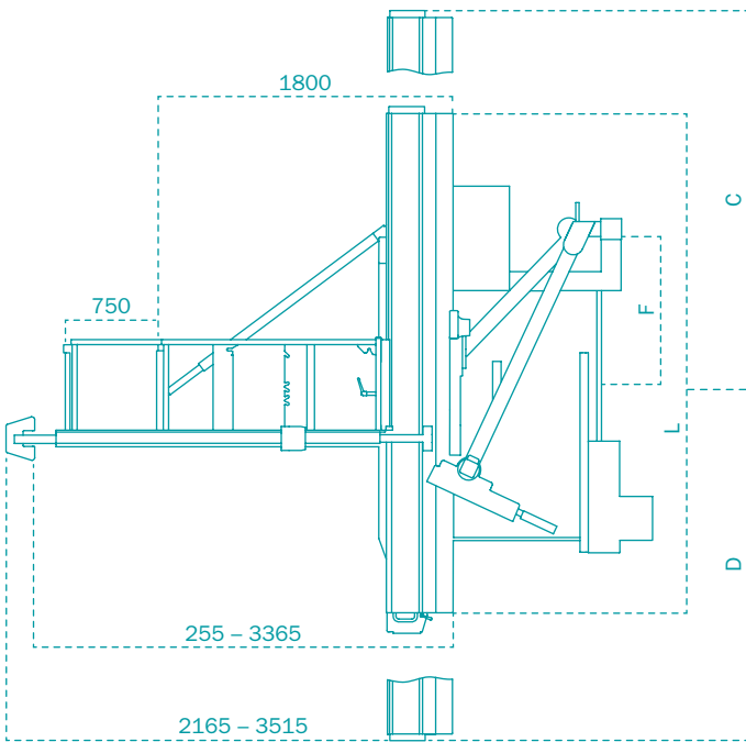
T75 | Draufsicht
