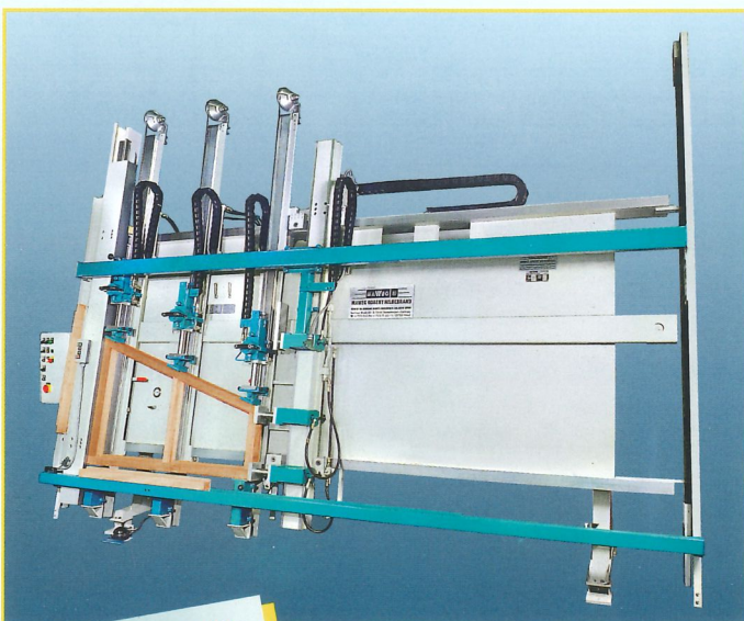
Quickomat U-Z mit Schrägfenstereinrichtung
