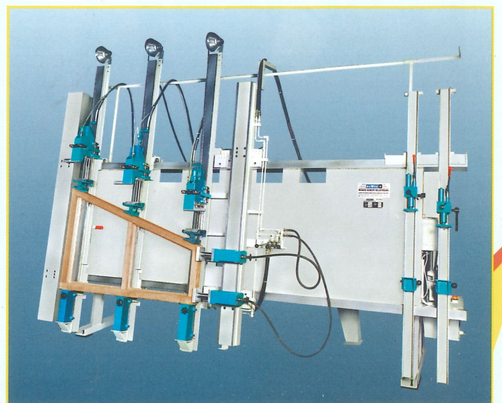
Rahmenpresse Euronova Z mit Schrägfenstereinrichtung
