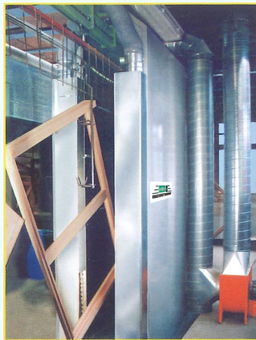
Einlauf in die Flutlackieranlage
