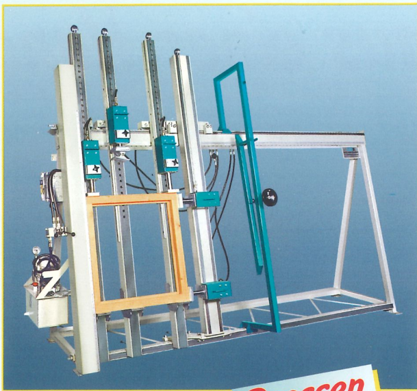
Rahmenpresse Euro Universal mit Niederhalter
