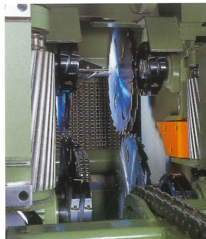
Doppelwellen-Kreissägenaggregat
