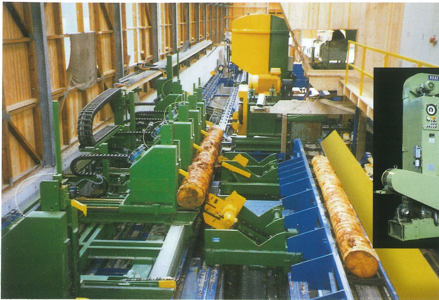
Blockbandsäge mit automatischer Beladung
