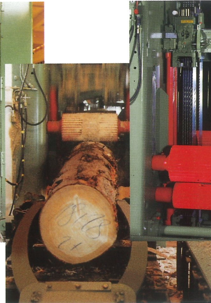
Breitenverstellung MULTI-BV
