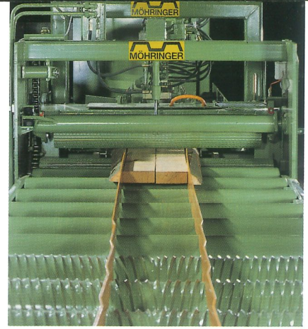
LamellenspreiBelabscheider
