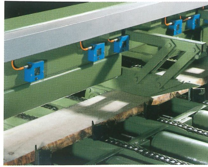
Automatischer Säumer mit Laservermessung
