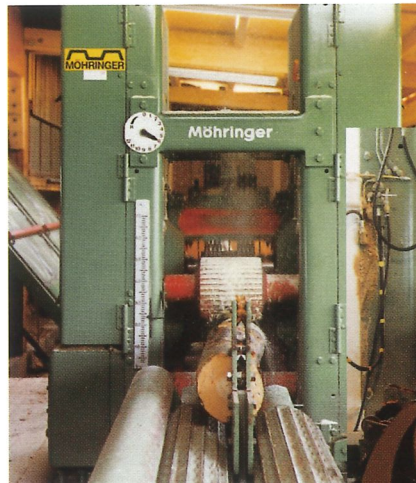
Gatter mit Schnelleinzug
