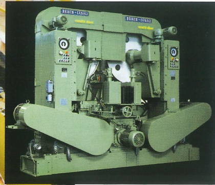
Vertikale Trennbandsäge
