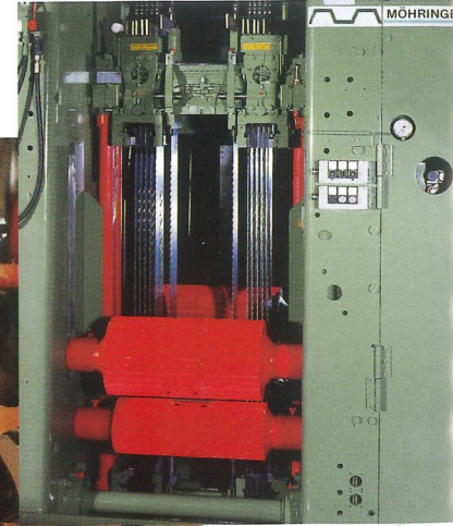
Breitenverstellung MULTI-BV
