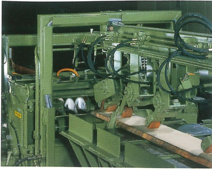
Positioniertisch
