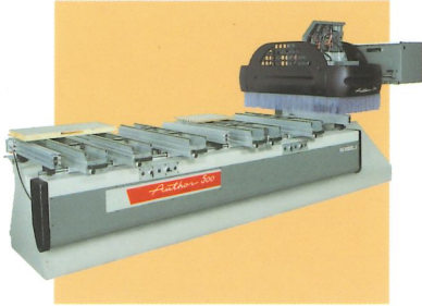
NC-gesteuertes Bohr- und Fräszentrum
