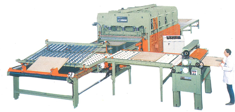
Linea di pressatura in ciclo continuo LCC Through feed press (end loading) LCC Ligne a plaquer en continu LCC Linea de prensado en ciclo continuo LCC Durchlaufpreßanlage LCC
