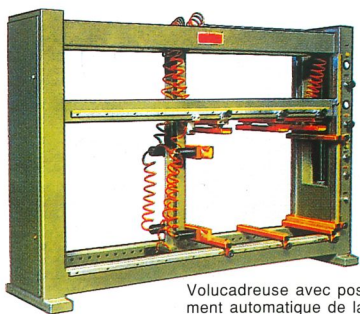
Strettoio per corpi di mobili con posizionamento automatico della trave tipo SMF/AUTOMATICO Carcass cramp with automatic positioning of the horizontal beam type SMF/AUTOMATICO
