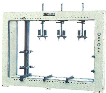
Strettoio per corpi di mobili SMF 26/16 Carcass cramp type SMF 26/16 Volucadreuse type SMF 26/16 Prensa neumatica para cuerpos de muebles SMF 26/16 Korpuspresse SMF 26/16
