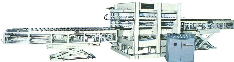
Impianto con carico e scarico automatico per la lavorazione del poliuretano Complete plant for poliurethane, automatic feeding and outfeeding Ligne en continu pour le poliurethane Linea con carga y descarga automatica especial para el poliuretano Anlage zur Bearbeitung von Polyurethan mit automatischer Beschickung und Entladung
