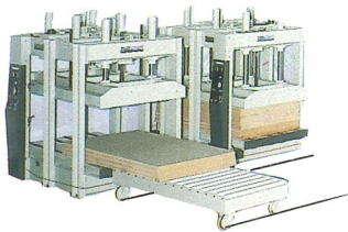
Impianto di pressatura automatico a freddo Automatic cold pressing system Ligne de pressage automatique a froid Instalacion de prensado en frio Automatische Kaltpreßanlage
