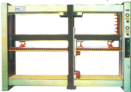
Strettoio per corpi di mobili autocontrante tipo SMF/SUPER Self setting carcass cramp type SMF/SUPER Volucadreuse automatique type SMF/SUPER Prensa neumatica para cuerpos de muebles con auto-centrado SMF/SUPER Selbstzentrierende Korpuspresse SMF/SUPER
