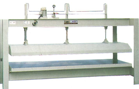
Pressa a freddo P 30/3 (disponibile anche con piani a caldo PCL 30/3) P 30/3 cold press (hot version too PCL 30/3) Presse a froid P 30/3 (disponibile aussi a chaud PCL 30/3) Prensa en frio P 30/3 (disponibile con platos calientes PCL 30/3) Kaltpresse P 30/3 (auch mit Heizplatten, Ausführung PCL 30/3)
