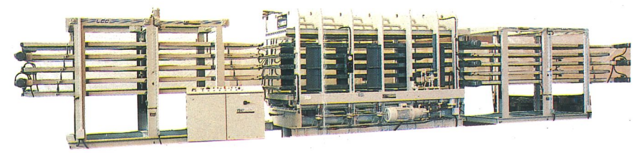
Linea di pressatura in ciclo continuo Multidaylight through feed press (end loading) Ligne a plaquer en continu Linea de prensado en ciclo continuo Durchlaufpreßanlage
