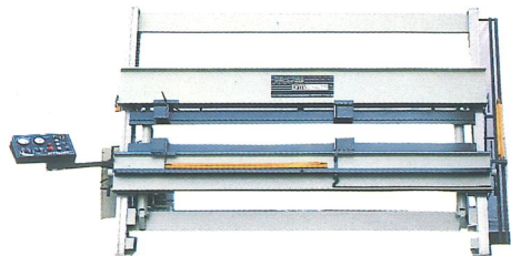
Strettoio SU/FUTURA a ricerca automatica Frame press SU/FUTURA with automatic positioning Cadreuse SU/FUTURA a recherche automatique Banco de armar con busqueda automatica de la madera SU/FUTURA Rahmenpresse SU/FUTURA mit automatischer Positionierung
