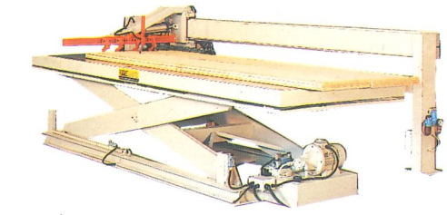
Piattaforma elevatrice con spintore pneumatico Lifting table complete with pneumatic pusher Plateforme elevatrice avec pousseur pneumatique Plataforma elevadora con empujador pneumatico Hebebühne mit pneumatischem Stößel
