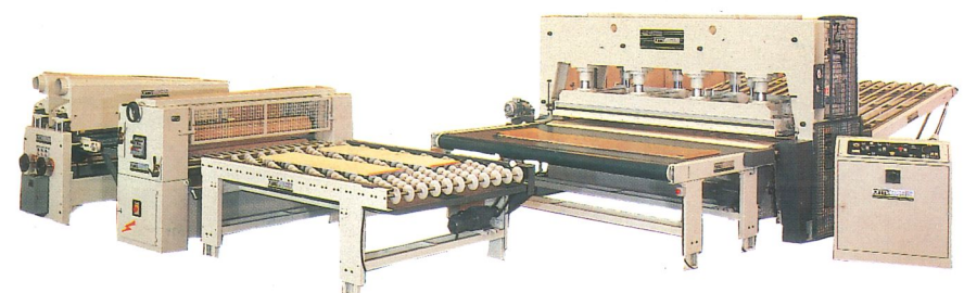
Linea di pressatura in ciclo continuo PCC Through feed press (side loading) PCC Ligne a plaquer en continu PCC Linea de prensado en ciclo continuo PCC Durchlaufpreßanlage PCC
