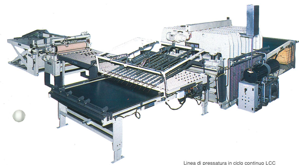
Linea di pressatura in ciclo continuo LCC Through feed press (end loading) LCC Ligne a plaquer en continu LCC Linea de prensado en ciclo continuo LCC Durchlaufpreßanlage LCC
