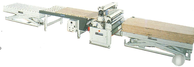
Impianto di pressatura automatico a freddo Automatic cold pressing system Ligne de pressage automatique a froid Instalacion de prensado en frio Automatische Kaltpreßanlage
