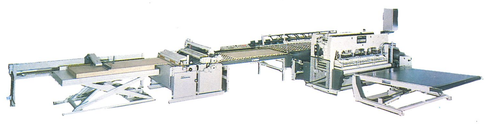
Linea di pressatura in ciclo continuo PCC Through feed press (side loading) PCC Ligne a plaquer en continu PCC Linea de prensado en ciclo continuo PCC Durchlaufpreßanlage PCC
