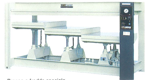
Pressa a freddo speciale Special cold press Presse a froid speciale Prensa en frio especial Sonderkaltpresse
