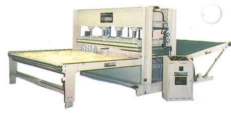
Linea di pressatura in ciclo continuo PCC/L Through feed press PCC/L (side loading) Ligne a plaquer en continu PCC/L Linea de prensado en ciclo continuo PCC/L Durchlaufpreßanlage PCC/L
