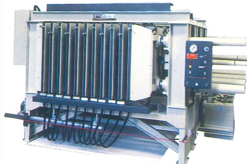
Presse per la lavorazione del poliuretano tipo PXE Presses for poliurethane type PXE Presses pour poliurethane type PXE Prensa para el poliuretano tipo PXE Presse Typ PXE zur Bearbeitung von Polyurethan
