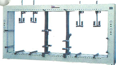
Strettoio per corpi di mobili a due stazioni di lavoro SMF 51/28 Two working stations carcass cramp type SMF 51/28 Volucadreuse a deux place de travail SMF 51/28 Prensa neumatica para cuerpos de muebles con 2 puestos de trabajo SMF 51/28 Korpuspresse SMF 51/28 mit 2 Arbeitsräumen
