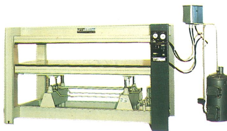
Pressa a caldo C/4 (disponibile anche con piani a freddo S/4) C/4 hot press (cold version too S/4) Presse a chaud C/4 (disponibile aussi a froid S/4) Prensa platos calientes C/4 (disponible con platos frios S/4) Heizplattenpresse C/4 (auch in kalter Ausführung S/4)
