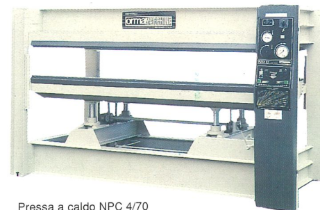
Pressa a caldo NPC 4/70 NPC 4/70 hot press Presse a chaud NPC 4/70 Prensa platos calientes NPC 4/70 Heizplattenpresse NPC 4/70
