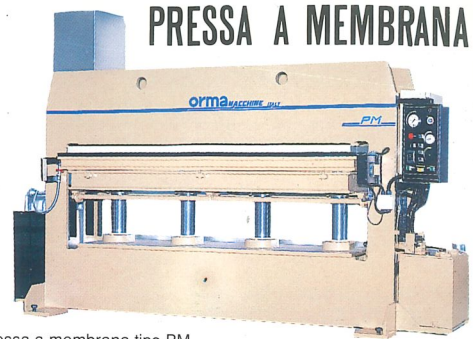
Pressa a membrana tipo PM Membrane press PM Presse a membrane PM Prensa a membrana tipo PM Membran-Formenpresse Typ PM
