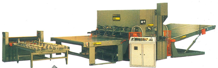
Pressa per l'incollaggio di listelli in automatico tipo PCS Edge-joining and veneering through-feed press PCS Ligne de panneautage et piacage en continu type PCS Prensa para la formacion de paneles alistonados en automatico PCS Presse zur Leistenplatten-Herstellung Typ PCS
