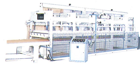
Linea di pressatura in ciclo continuo LCC Through feed press (end loading) LCC Ligne a plaquer en continu LCC Linea de prensado en ciclo continuo LCC Durchlaufpreßanlage LCC
