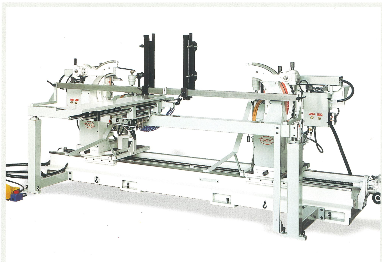
► NS21 con cargamento/scaricamento automatico modelo CS ► NS21 with hopperfeeder model CS ► NS21 mit automatischem Beschickungsmagazin Model CS ► NS21 avec chargeur automatique mod. CS ► NS21 con cargador automatico mod. CS
