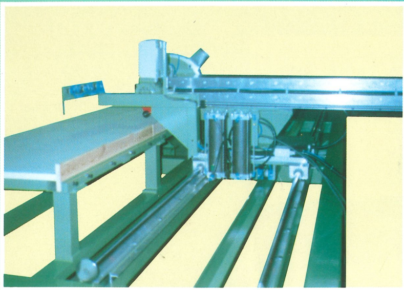
◀ Fahrbare-Platten- Aufschneid-Säge PLSE-A; Schnittlänge = 1250 mm von Hand verschiebbar, Anzeige mit Digital-Meßeinrichtung. Die gesamte Säge fährt in der Halle auf Schienen.
