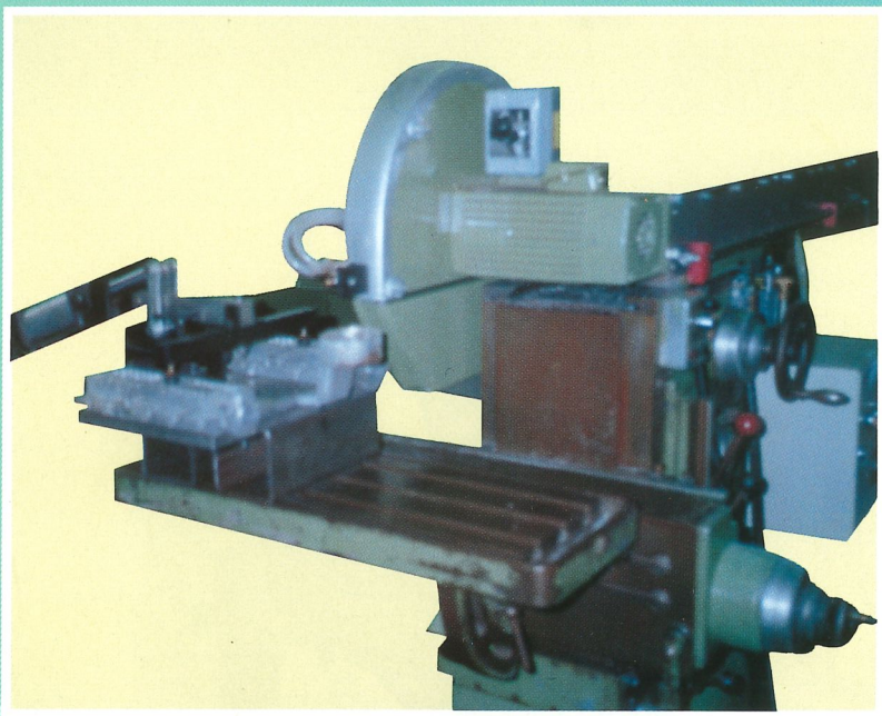
▲ Aufbau einer PLSE-Einheit auf alte Fräsmaschine. Bearbeitung von Alu-Kokillen-Gußteilen.
