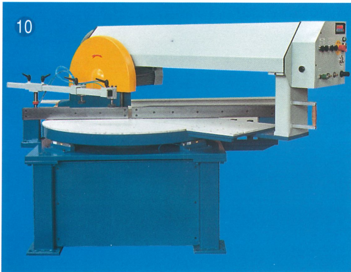
10 Präzisions-Gehrungssäge für universellen Einsatz in der Leichtmetall-, Kunststoff- und Holzverarbeitung.
