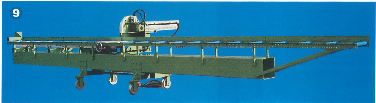
9 Säge für Regallager auf Schienenfahrwerk quer verfahrbar. Aufgabeseite rechts 6,5 m, Fertigungsseite links 3,5 m mit Digitalanschlag.
