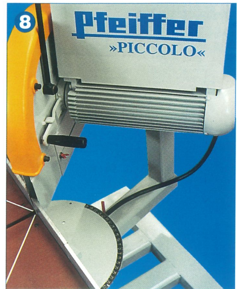
8 Detail: Große, gut ablesbare Gradskala am Gehrungssägetisch (GSE) – verstellbarer unterer Sägeschutz.
