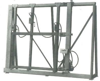
Hydraulik- oder Pneumatik-Rahmenpresse für den Mittelbetrieb
