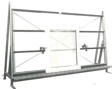
Montagevorrichtungen für Rahmenmontage
