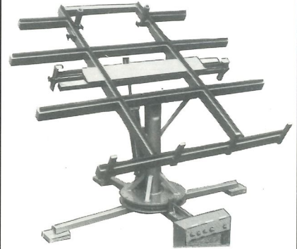
Pneumatik-Dreh-Kipptisch
