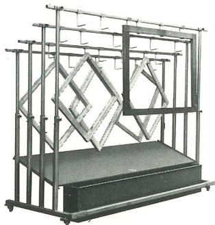
Tauchanlage mit Aufhängevorrichtung oder mit Aufstellvorrichtung
