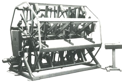
Etagen-Verleimsterne, auch als Sonderanfertigung
