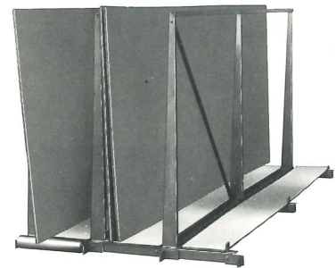
Plattenregal im Baukastensystem
