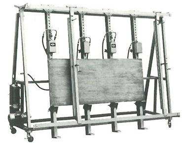
Fugenverleimpresse, stabil, stehend oder fahrbar
