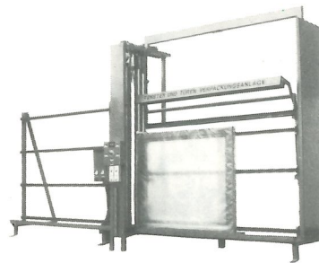
Folien-Verpackungsstand für Fenster, Türen u. Elemente
