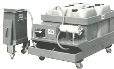
Filter- und Pumpstation für alle Tauchflüssigkeiten
