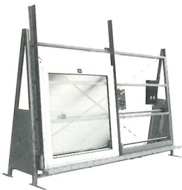
Vollpneumatik-Verglasungspresse und Kontrollstand
