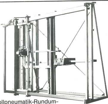
Vollpneumatik-Rundum- fräsmaschine für die Holzfenstersanierung. Umrüstung von Einfach- auf Doppelverglasung
