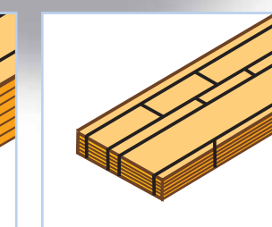
Längs- und Querschneiden von Plattenpaketen
