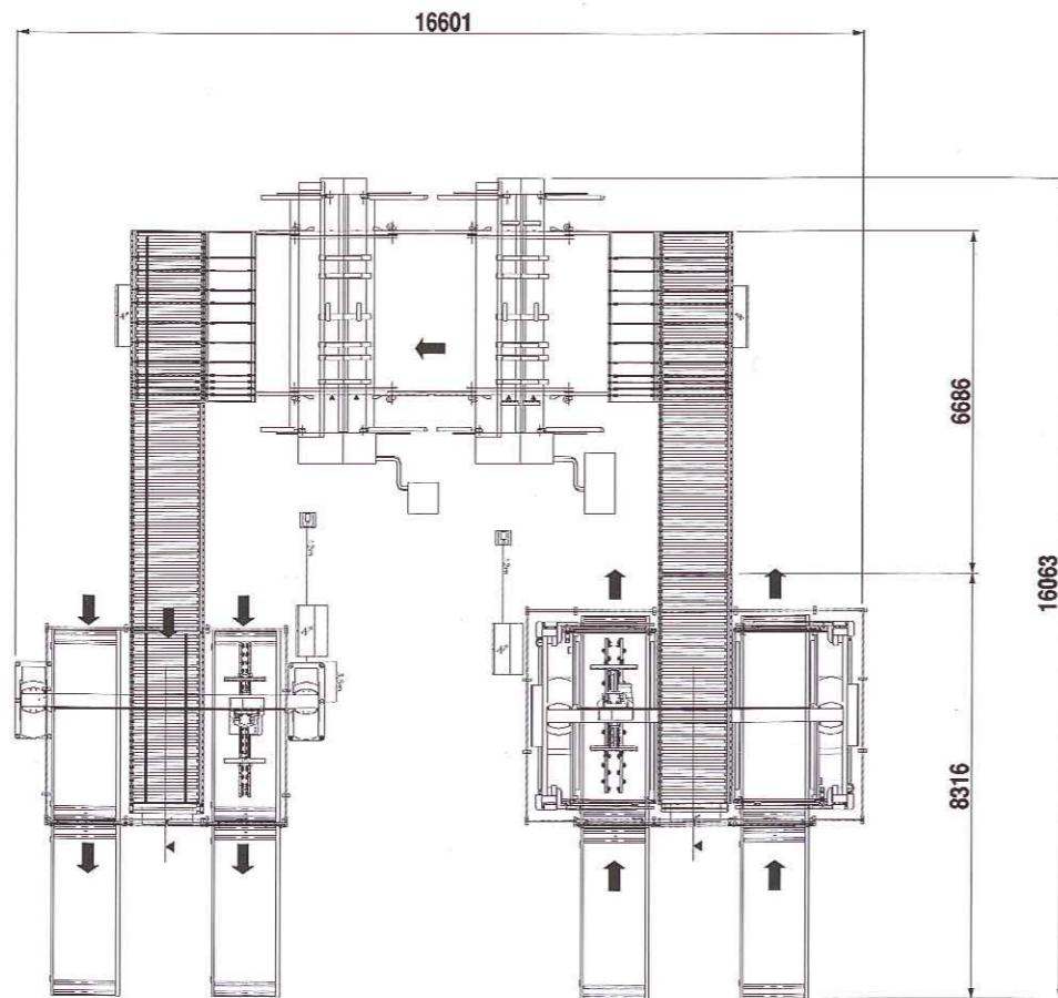
Bohrstraße mit Beschickung/Abstapelung Winner und Winkelübergaben.
