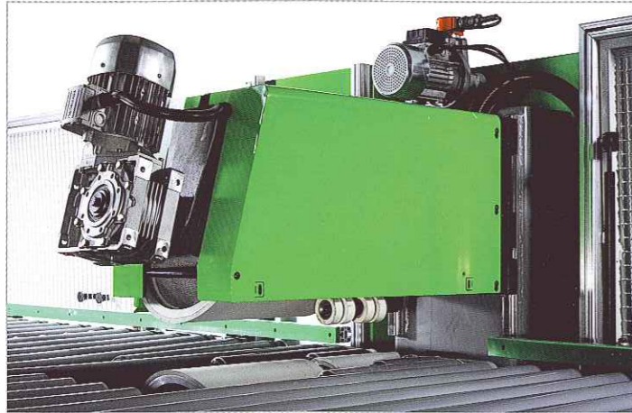
Detail der Drehstation mit Kegeln.
