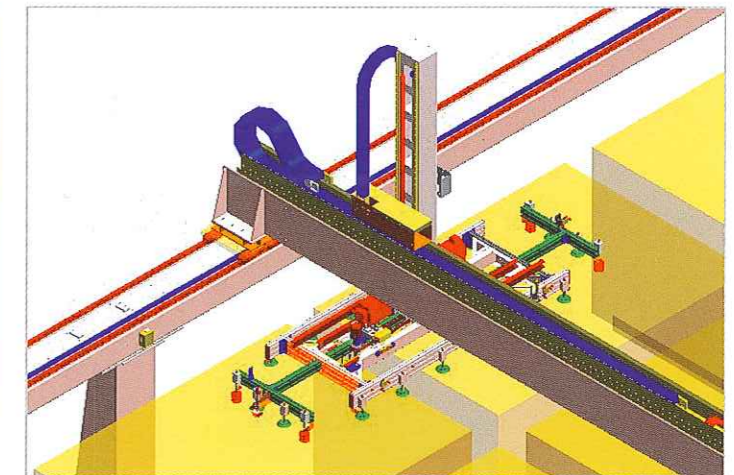
Automatischer Saugrahmen mit teleskopischer Öffnung.
