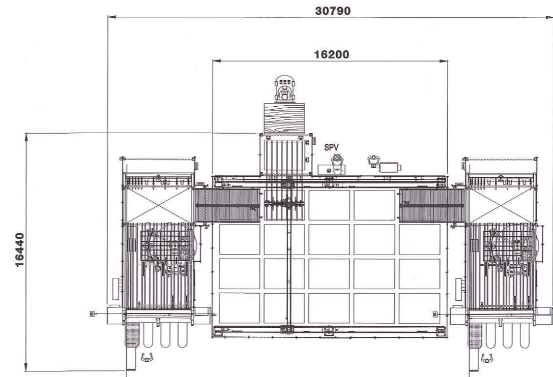
Automatisches Lager für Plattenaufteilstrasse.
