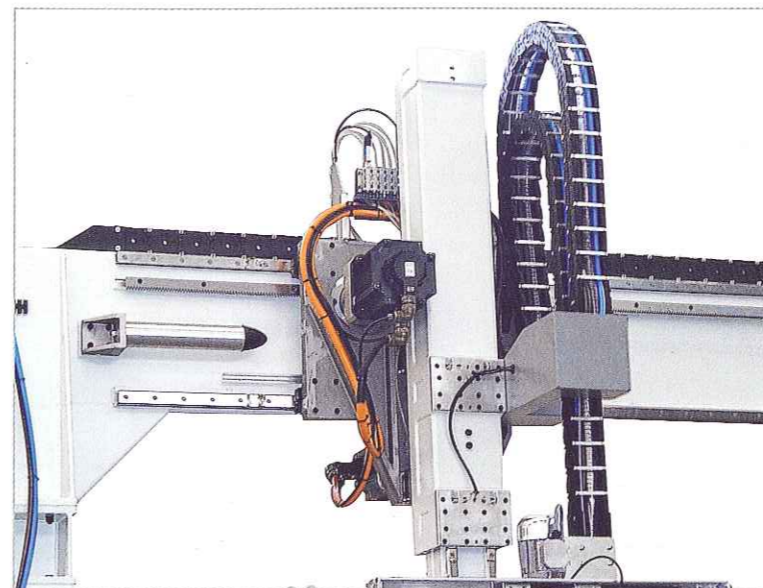
Saugrahmen mit teleskopischer Säule.
