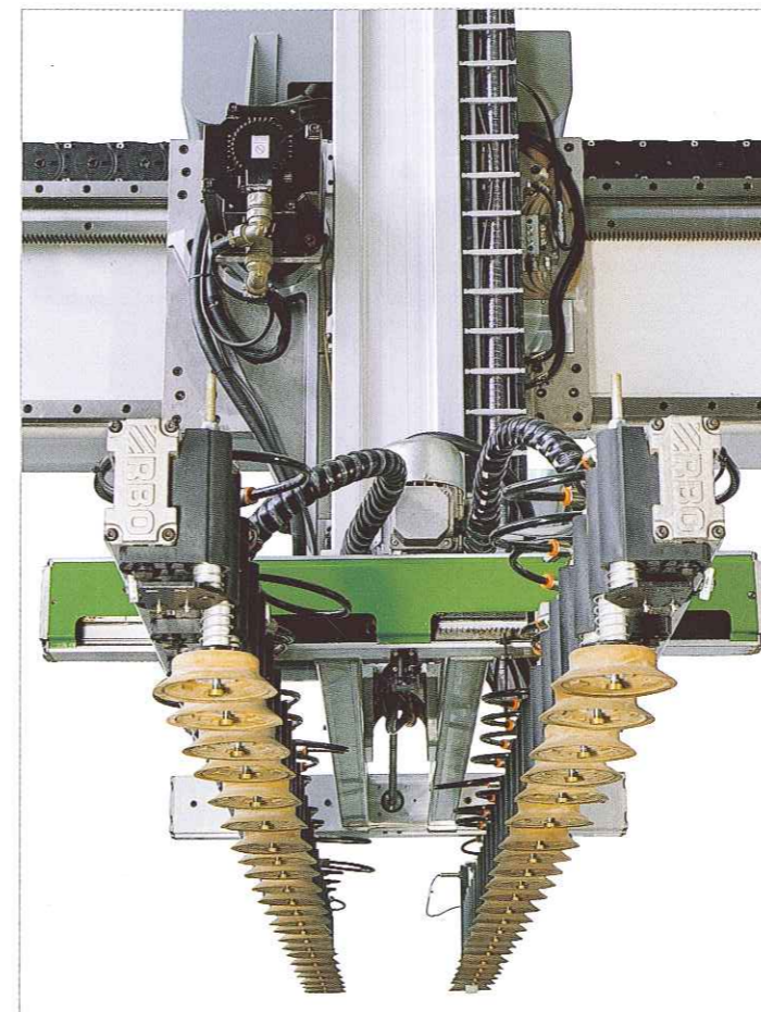
Automatisch einstellbare Saugerrahmen.
