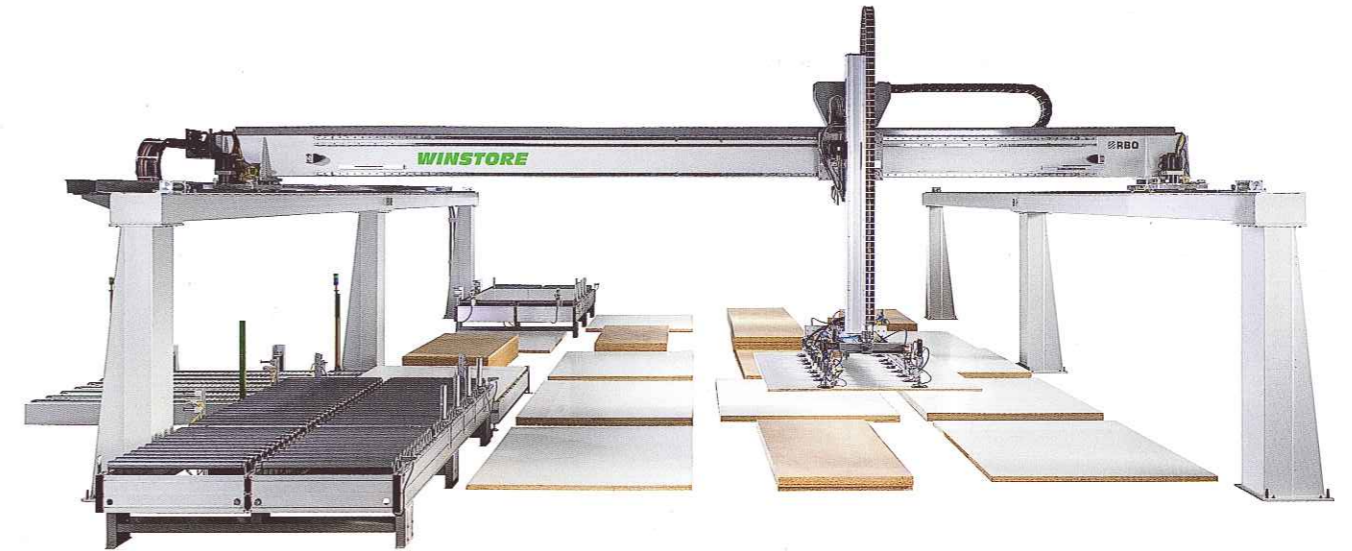
Winstore 3D: 3-Achsen automatische Picking-Lagerungsanlagen.
