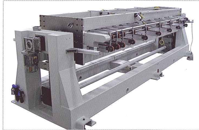
Kippvorrichtung mit Riemen für Fertigungslinien zur Drehung von Platten um 180° in Querrichtung oder als Durchlauförderer. 20 Zyklen/min in einzelreihe und 13 Zyklen/min in doppelreihe.
