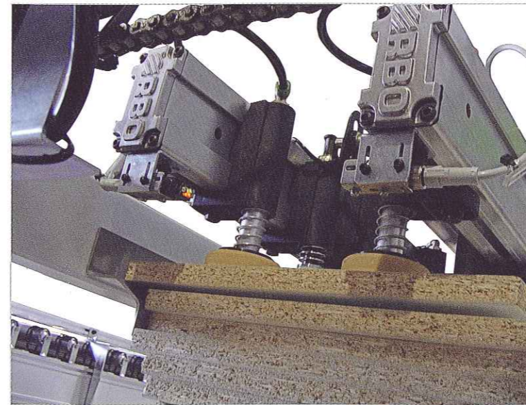
Mechanischer Plattentrenner.
