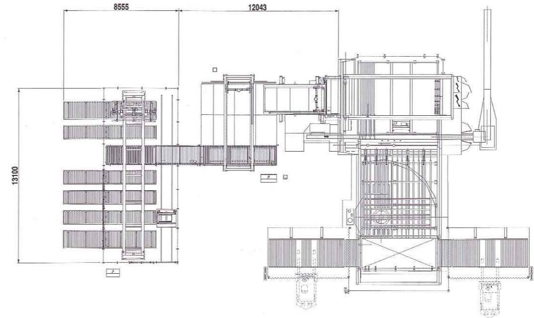
Plattenaufteilstraße mit Längsabziehvorrichtung, Querschubvorrichtung und Abstapelung Lifter 2T.
