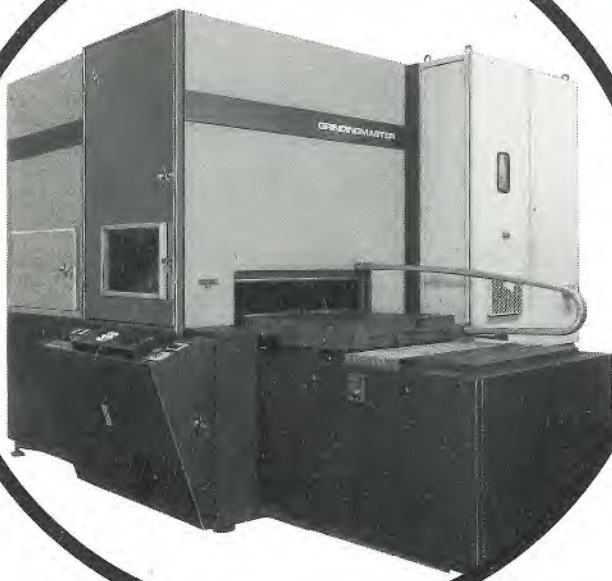
Hi-Gee Hochleistungsplanschleifmaschine mit 135 kW-Hauptmotor.
