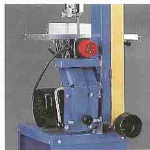
Die Schnittgeschwindigkeit läßt sich stufenlos den Erfordernissen anpassen.
