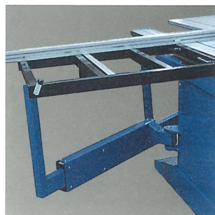
Der große Quertisch mit dem neuen Teleskoparm als Zubehör ermöglicht optimale Schnittergebnisse.
