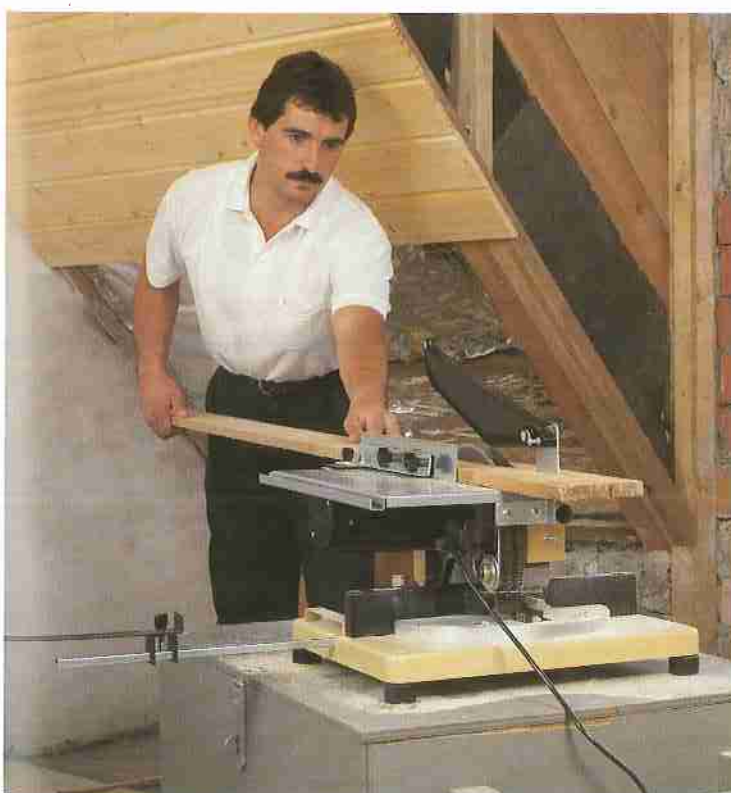
Bild oben: Gehrungschnitt mit der scheppach KG 250
