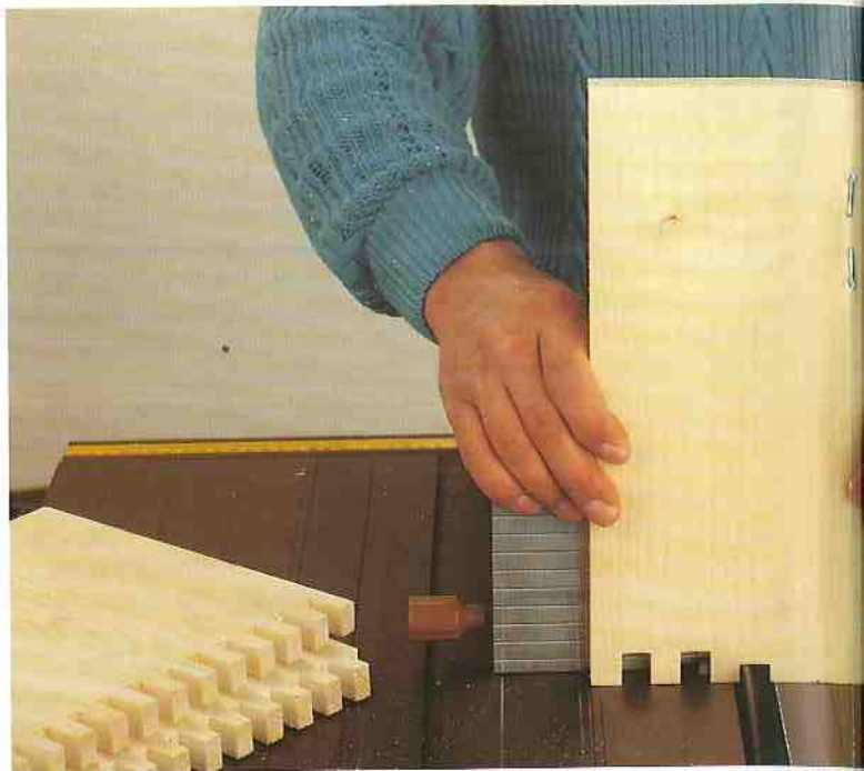
Zinkenschneid-Einrichtung ▲
