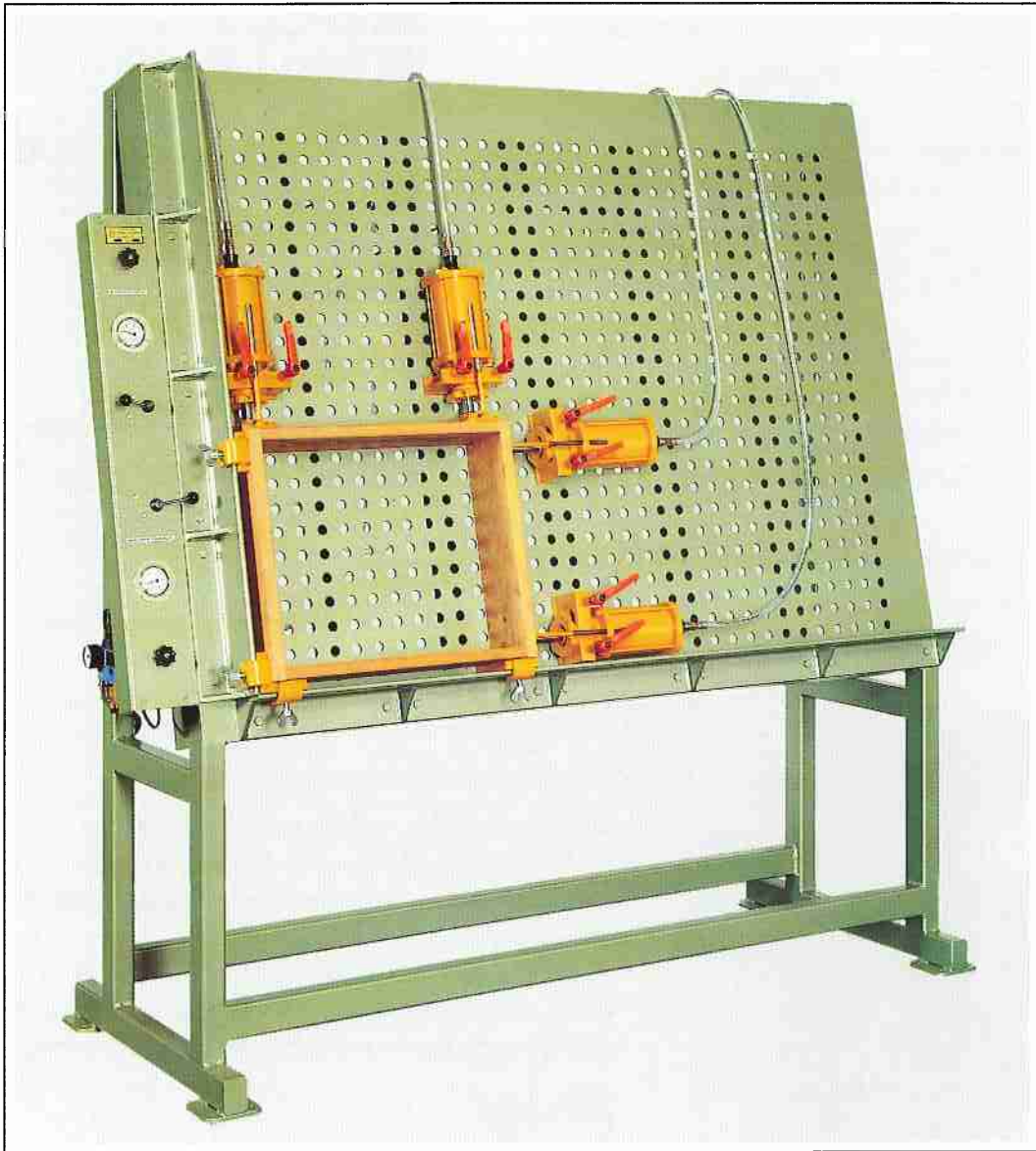
Tischpresse mit Druckluftzylinder in schräger Ausführung
