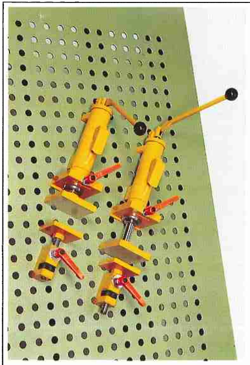
Handhydraulische Spannelemente und Gegenböcke in schwenkbarer Ausführung
