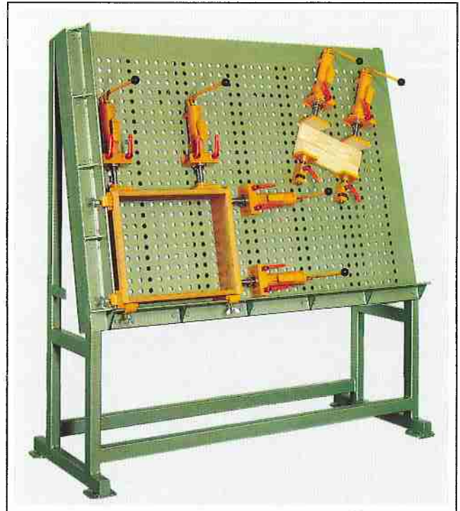
Tischpresse mit handhydraulischen Spannelementen in schräger Ausführung
