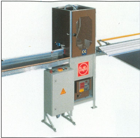
Armierungsschrauber 2757
