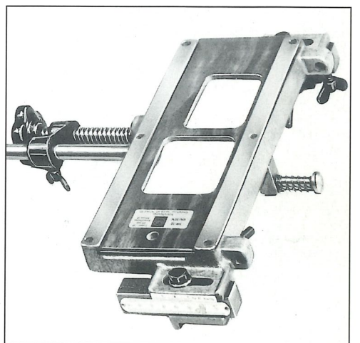
Fräsrahmen 118
