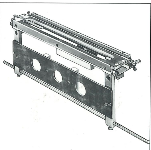
Fräsrahmen 114
