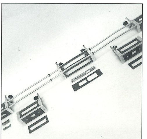
Anschlagsatz 180
