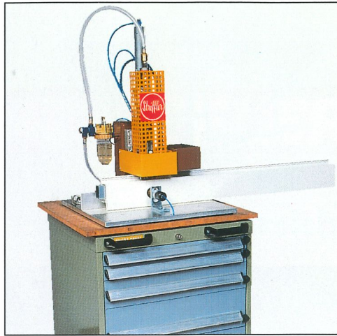
Armierungsschrauber 2954
