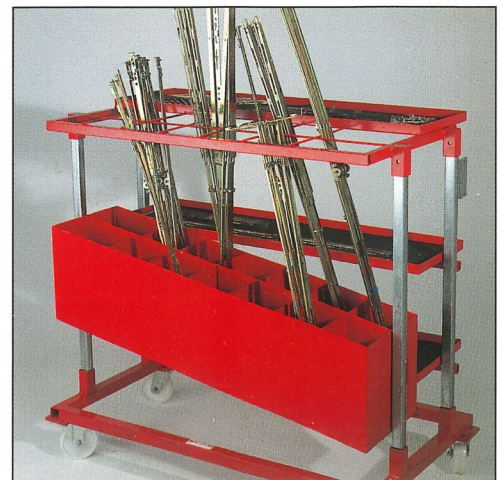
Transport-Beschlagwagen TBW
