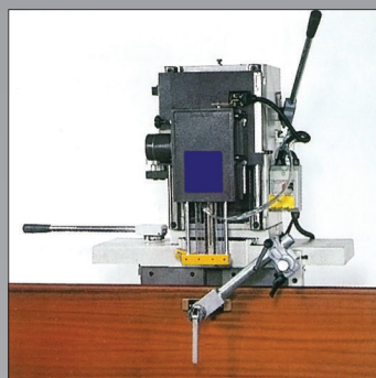
Macchina predisposta per lavorazione di porte Machine set for door working Machine predisposée pour l'usinage de portes Maquina predispueta para la elaboracion de puertas
