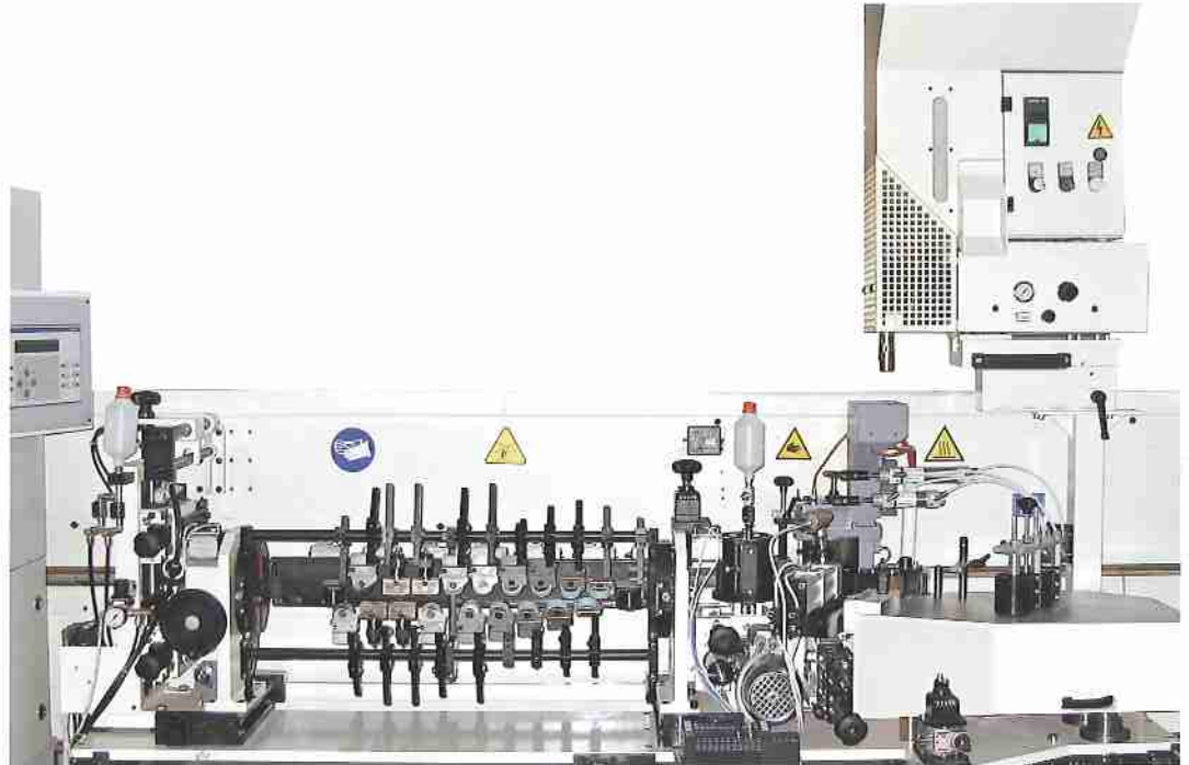
Gruppo incollaggio soffforming Soffforming gluing unit Grupo encolador soffforming
