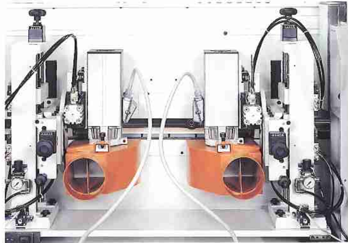
Gruppo toupie Grooving unit Grupo tupí para ranuras
