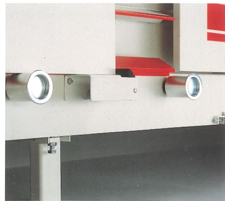
Auflagerollen mit Werkstück-Arretierung
