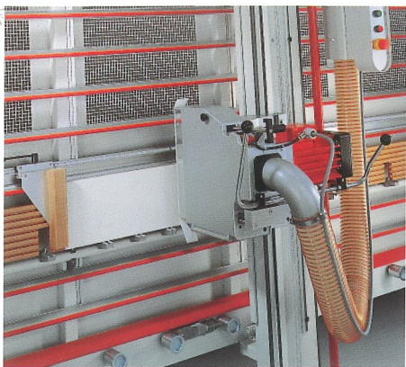
Grossflächiger Längsanschlag
