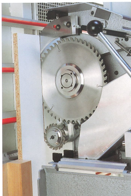
Vorritz-Sägeaggregat VSA
