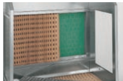
Die Filtermedien, Vor- und Feinfilter, sind bei Bedarf mit wenigen Handgriffen gewechselt.
