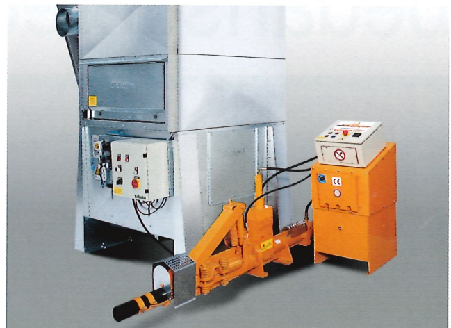
■ VACOMAT-S mit angebauter Schuko-Brikettierpresse, Baureihe Compacto, Typ 800 S
