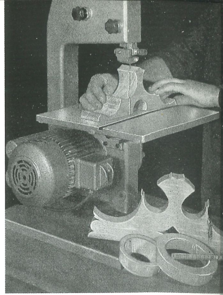
Auftrennen eines Kantholzes in dünne Brettchen Sagen geschweifter Konturen
