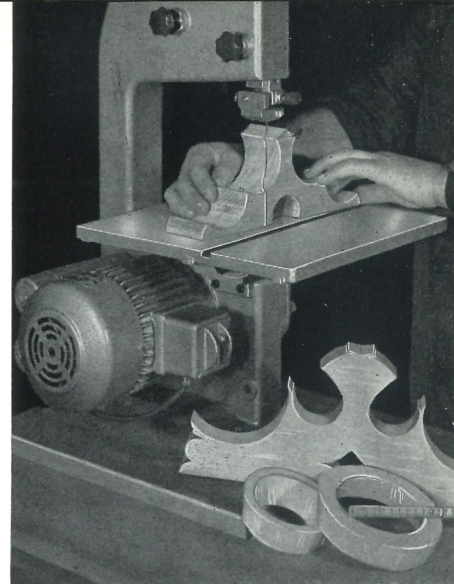
Auftrennen eines Kantholzes in dünne Brettchen Sägen geschweifter Konturen
