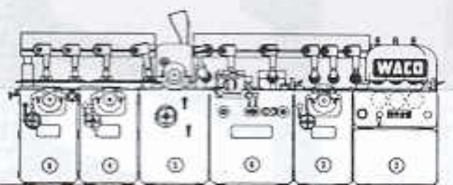
6-spindlig profilhyvel med huvudmatarverk.
