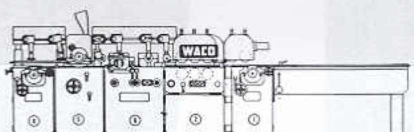
5-spindlig riktlisthyvel.
