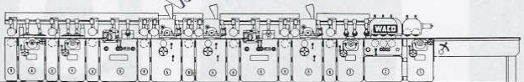
11-spindlig rikt- och profilhyvel med genomgående matning för korta arbetsstycken. 16 övre och 11 undre drivna valsar. Specialkombination för högproduktiv hyvling av fönsterämnen. Max. matningshastighet 50 m/min.
