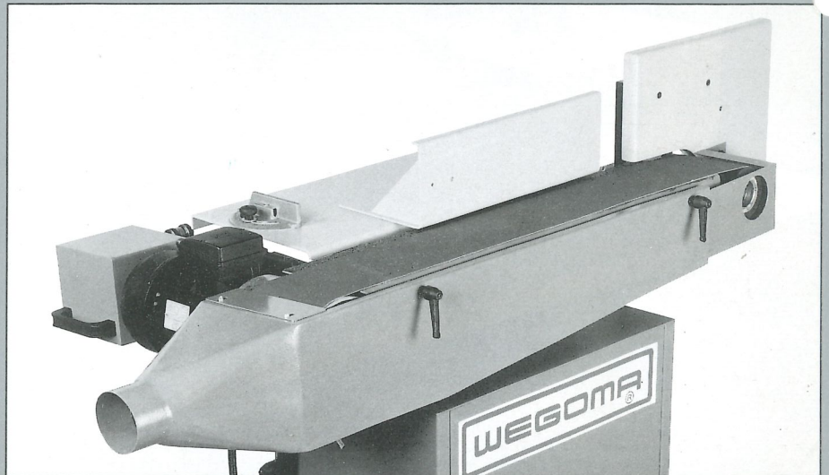
△ Schleifeinheit geschwenkt 180°
