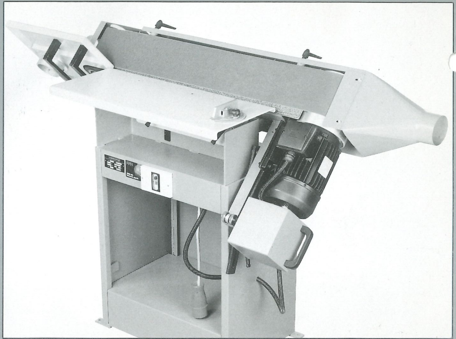
△ Schleifeinheit geschwenkt 45°
