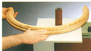
Rundsleifen an der Bandspannwalze
