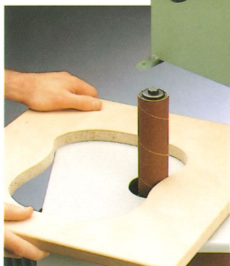
Selbst Werkstücke mit Innenausschnitt sind sauber zu schleifen
