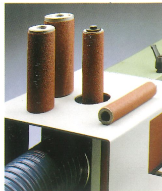
Serienmäßig mit 4 wechselbaren Schleifhülsen - nach Bedarf aufsteckbar
