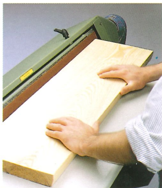
Präziser Kantenschliff durch 90° schwenkbares Aggregat
