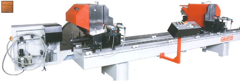
Doppelgehrungssäge DS 120 Double Mitre Saw DS 120 Tronçonneuse double DS 120
