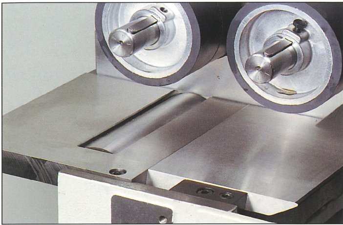
Verstellbarer Auslauftisch nach der unteren Profilierspindel. Schnell Rüsten. Keine Einschläge.
