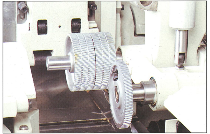
Teleskop-Pendelwelle gegenüber der linken Spindel. Schnell und stufenlos von schmalen auf breite Werkstücke einstellbar.
