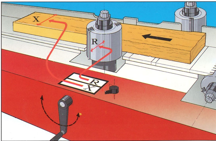
Weinig DigiSet für linke und obere Spindel. Werkzeug über digitale Doppelanzeigen direkt einstellbar. Fertigmaß in Breite und Dicke stets ablesbar.
