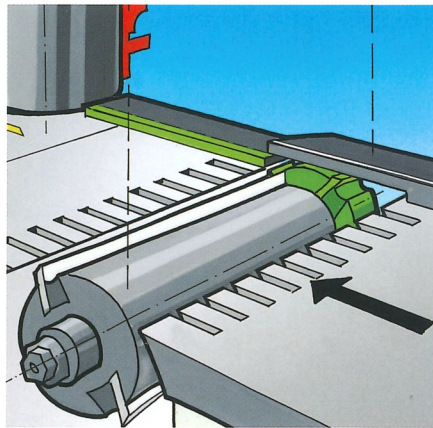
Abrichtspindel mit Falzfräser und geschlitzte Tischplatten: Präzision beim Abrichten und Fügen, Lärmschutz.
