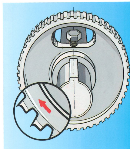
Spezialverzahnung der Vorschubwalzen verringert Eindringtiefe ins Holz. Gehärtet und verchromt. Selbstreinigend. Weinig Patent!
