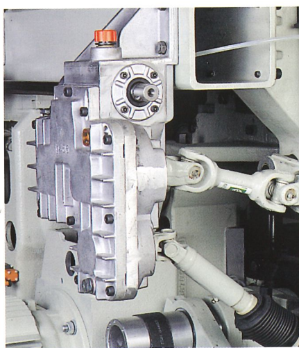
Kettenloser Kardanvorschub präzise, robust, langlebig und nahezu wartungsfrei!
