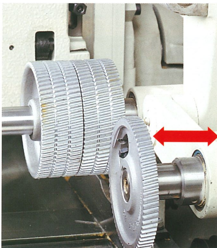
Teleskop-Vorschubwalze gegenüber der linken Spindel. Schnell und stufenlos von schmalen auf breite Werkstücke einstellbar.
