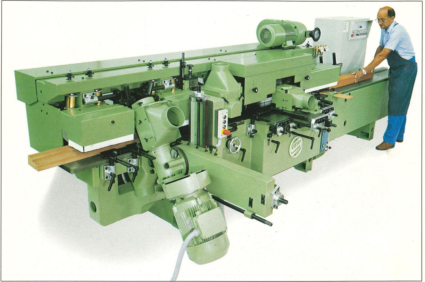
▲ La Unimat en la fabricación de ventanas: ¡Breves tiempos de preparación para pequeñas series!
