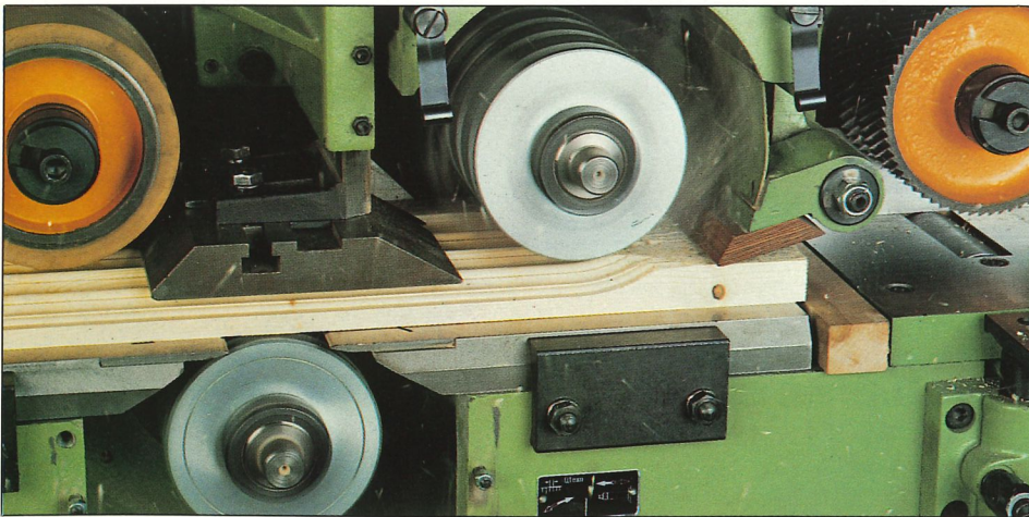
▲ He aquí algunas razones del éxito de la Unimat: Husillos de trabajo de alta precisión. Sólidas sujeciones. Sólidos prensos y guías. Pesada construcción de fundición. Sistema de avance perfectamente concebido. La técnica de Weinig.
