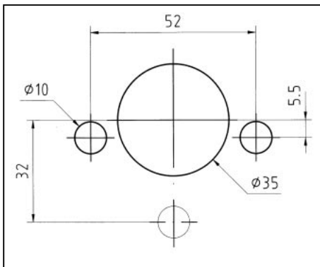
Bohrbild für Topfbänder
