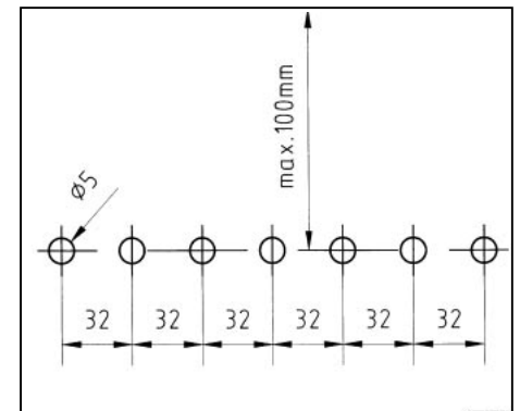
Bohrbild für Lochreihe
