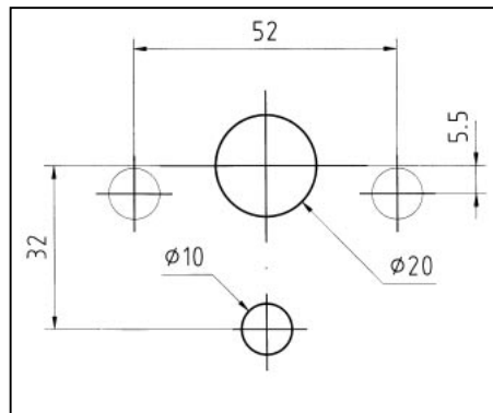
Bohrbild für Systemverbinder
