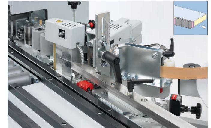
Olepovací agregát + přítlačná zóna
