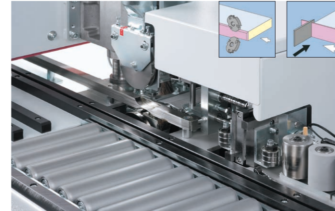
Kapovací agregát + frézovací agregát
