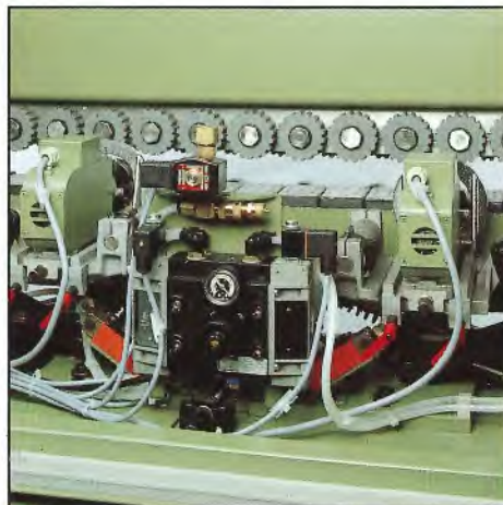
Formfräs- aggregat 4805
