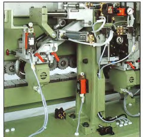
Formfräs- aggregat 4810
