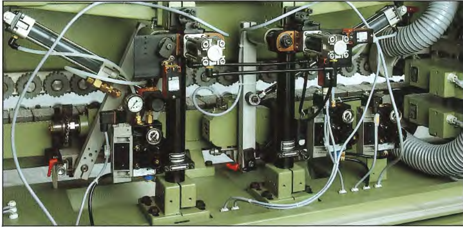
Kappaggregate 3150 und 3200
