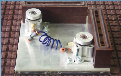
Ventose speciali per pezzi angolari dotata di pistoncini di riferimento a scomparsa.
