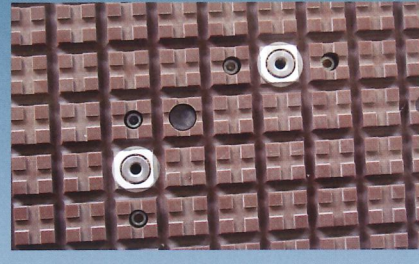
Particolare piano di lavoro in LPM quadrettato con pistoncini di riferimento parti ad angolo a scomparsa pneumatici e boccole con guarnizioni in gomma apribili con il semplice uso della calamita in dotazione al corredo
