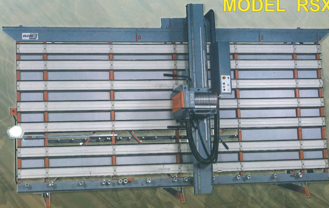
PODCINAK OBROTOWY
