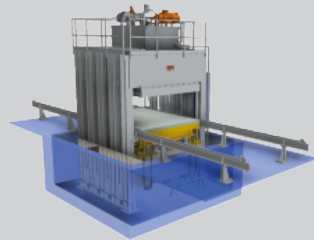
Presse zur Herstellung von Großformbauteilen Press for the production of big-sized molded parts
