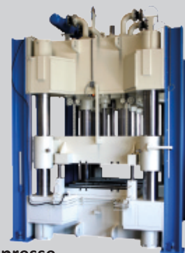
Kaschier-/Stanzpresse Laminating-/punch press
