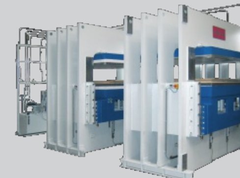
Pressenlinie zur Herstellung von Halbzeugen Pressing line for semi finished products
