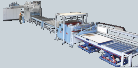
Durchlaufpresse für Plattenproduktion Feed-through press for board production
