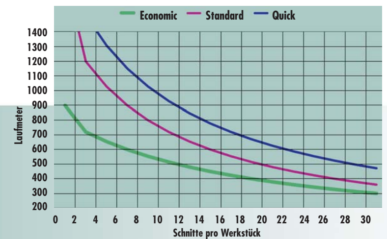
Leistungsdiagramm
