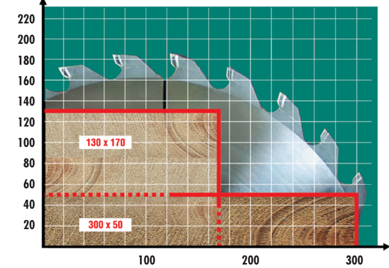
Schnittdiagramm
