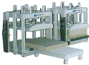
Impianto di pressatura automatico a freddo Automatic cold pressing system Ligne de pressage automatique a froid Instalacion de prensado en frio Система автоматического холодного прессования
