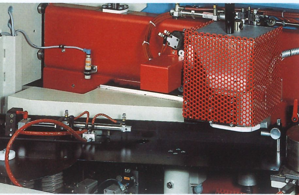
Maschineneinlaufseite mit untenliegendem Schnellheizbecken und Automatikmagazin
