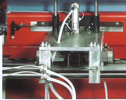
Maschineneinlaufseite mit untenliegendem Schnellheizbecken und Automatikmagazin
