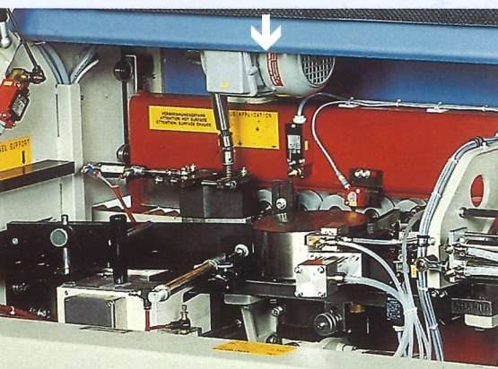
Maschineneinlaufseite mit untenliegendem Schnellheizbecken und Automatikmagazin
