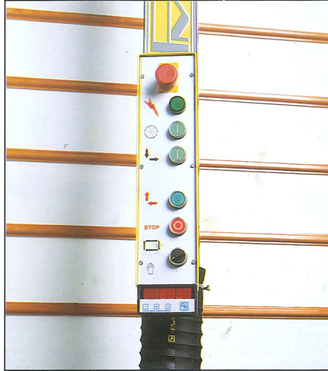
SVP 950 A Pulsantiera con visualizzatore elettronico quote orizzontali (optional) . / Switch-board with electronic measuring system of horizontal cuttings (optional) / Schalttafel mit Digitalanzeige für waagr. Schnitte (auf Wunsch) . / Teclado de mando con sistema de medición electrónico por los cortes horizontales (optional) / Tableau de commande avec lecture digitale électronique pour les découpes horizontales (optional) .
