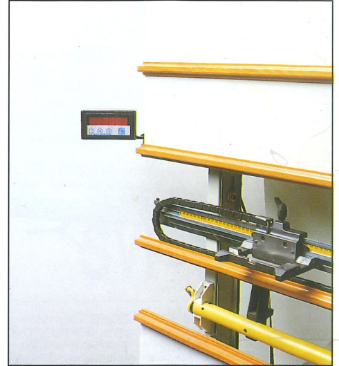
Visualizzatore elettronico quote verticali (optional) . Electronic measuring system of vertical cuttings (optional) . Digitale Massanzeige für senkrechte Schnitte (auf Wunsch) . Sistema de medición electrónico por los cortes verticales (optional) . Lecture digitale électronique pour les découpes verticales (optional) .
