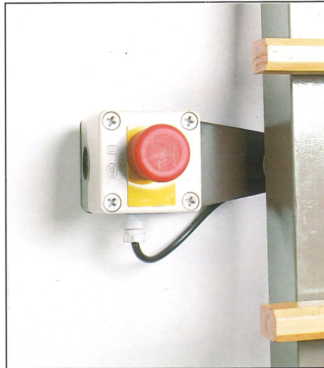
SVP 950 A Emergency-stop à gauche du châssis (standard) .
