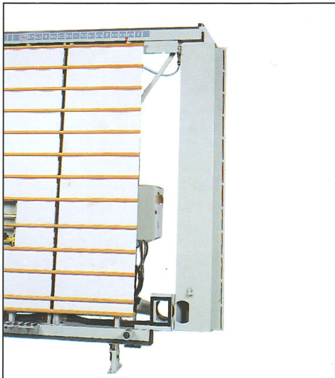
Sistema d'aspirazione "ECO" (optional). - Dust exhaust - ECO System (optional). - Absaugsystem ECO (auf Wunsch). Sistema d'aspiracion ECO (optional). - Systeme d'aspiration ECO (option).
